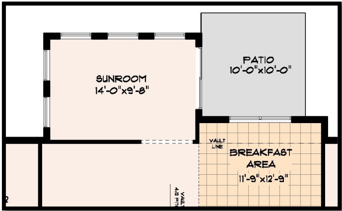
OPTIONAL SUNROOM
